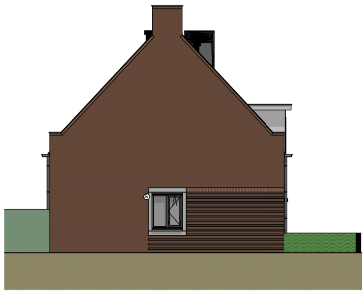
zijgevel oost
